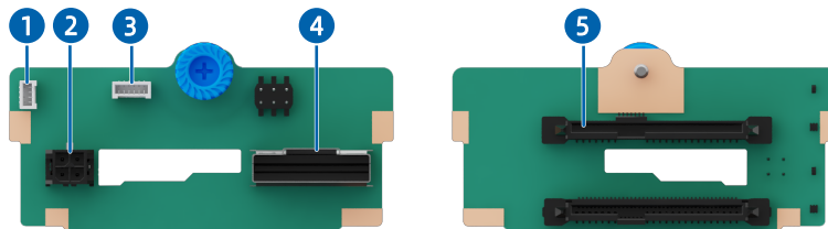
图 5-63 2 × 2.5 英寸硬盘配置 (2 × NVMe) 背板
