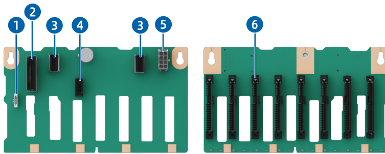
图 5-60 8 × 2.5 英寸硬盘配置 (6 × SAS/SATA&2 × SAS/SATA/NVMe) 背板
