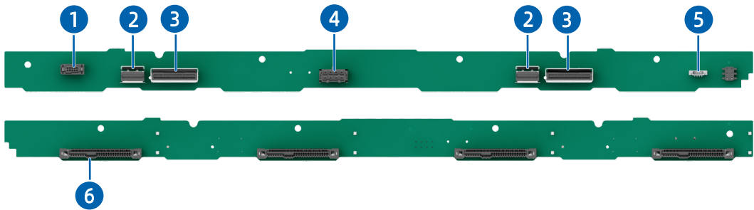
图 5-54 4 × 3.5 英寸硬盘配置 (4 × SAS/SATA/NVMe) 背板
