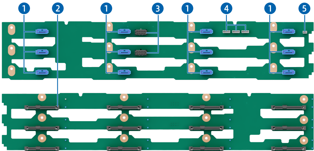
图 5-55 12 × 3.5 英寸硬盘直通配置 (12 × SAS/SATA) 背板
