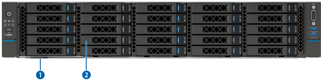
图 5-4 前面板外观
