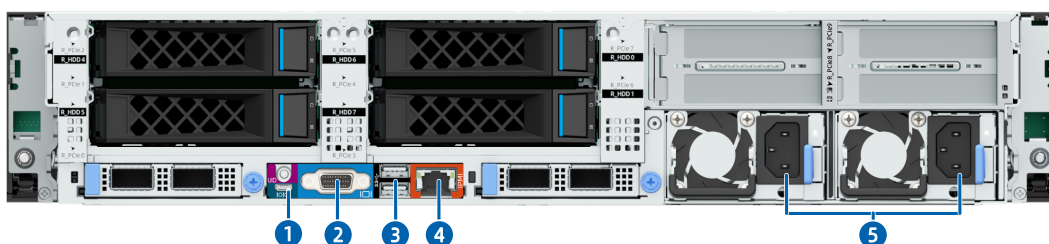
图 5-23 后面板接口
