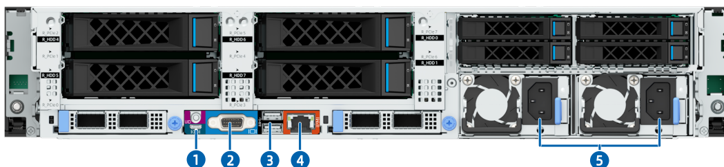
图 5-22 后面板接口
