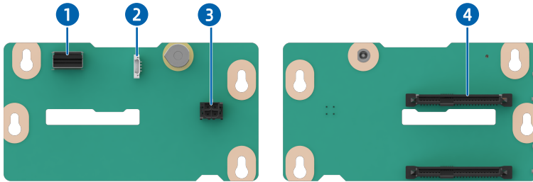
图 5-62 2 × 3.5 英寸硬盘配置 (2 × SAS/SATA) 背板
