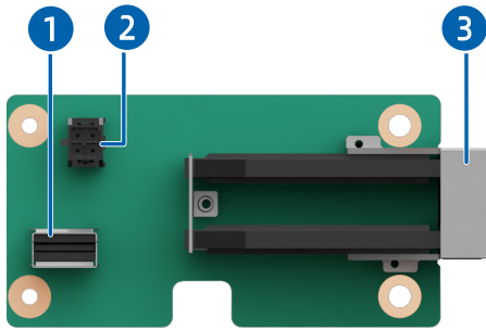
图 5-65 2 × M.2 硬盘配置背板
