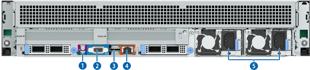
图 5-24 后面板接口
