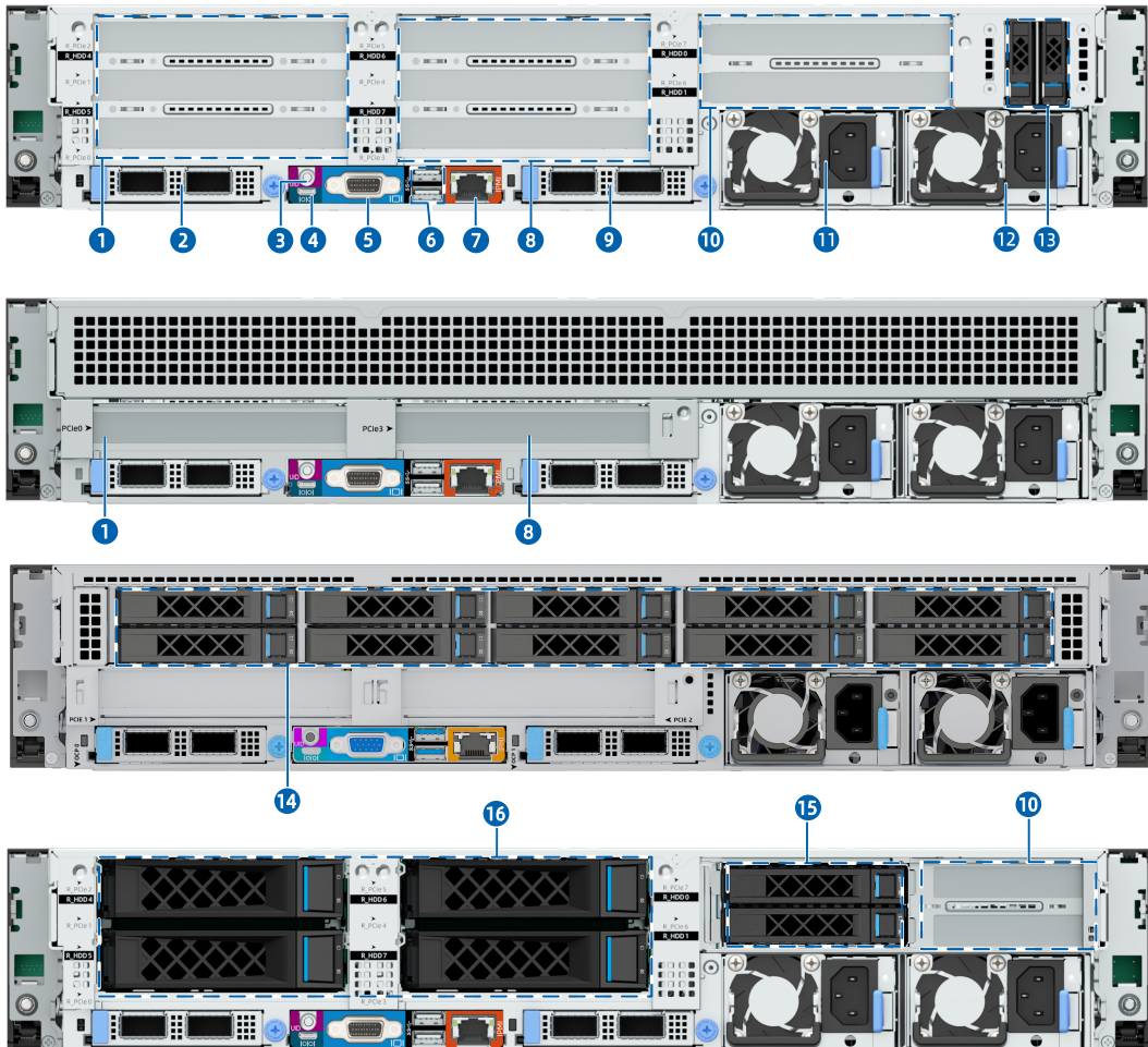
图 5-16 后面板外观
