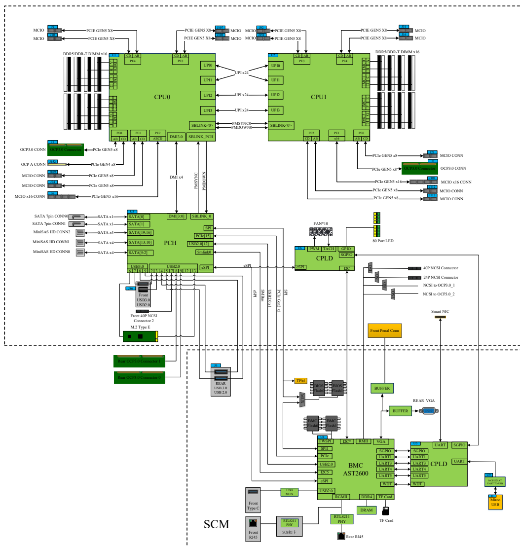
图 4-1 逻辑结构
