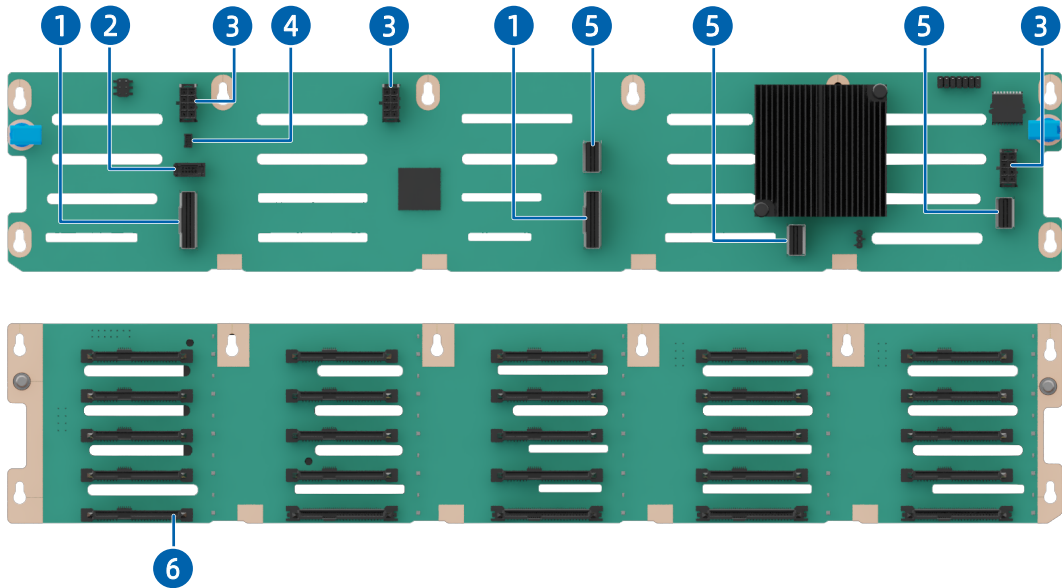
图 5-58 25 × 2.5 英寸硬盘配置 (21 × SAS/SATA&4 × SAS/SATA/NVMe) 背板
