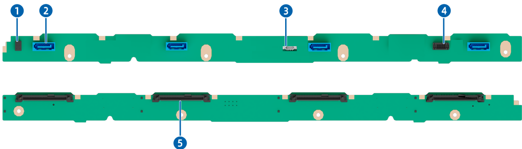
图 5-53 4 × 3.5 英寸硬盘配置 (4 × SAS/SATA) 背板
