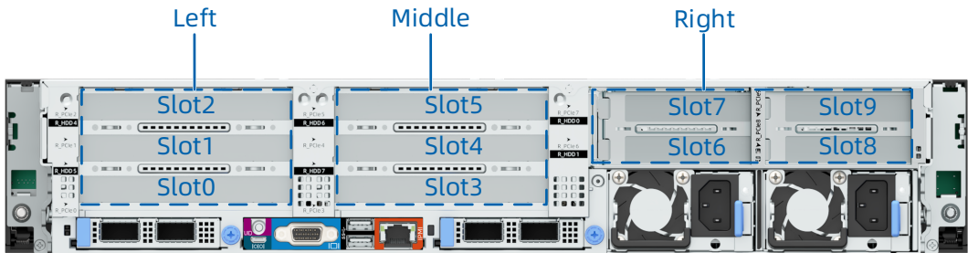
图 5-43 PCIe 插槽-10PCIe 配置
