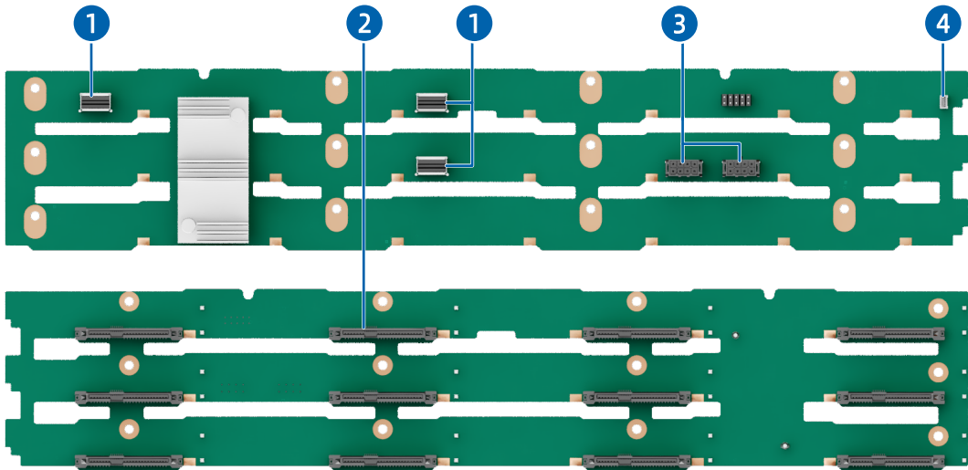
图 5-56 12 × 3.5 英寸硬盘配置 (12 × SAS/SATA) 背板
