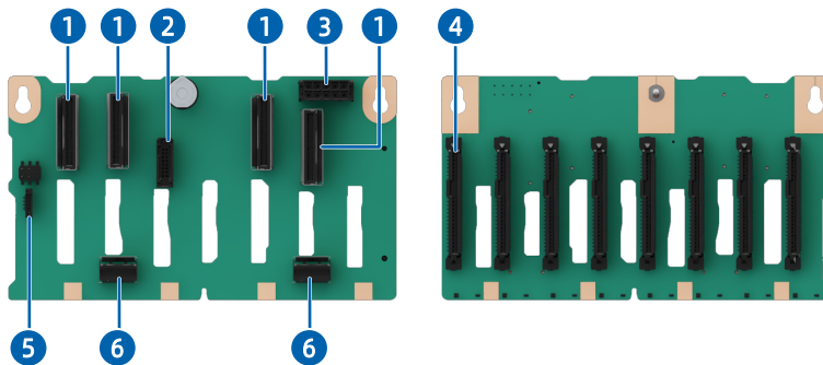
图 5-59 8 × 2.5 英寸硬盘配置 (8 × SAS/SATA/NVMe) 背板
