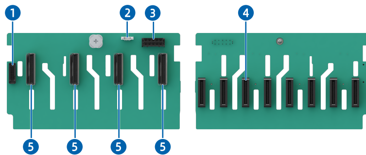
图 5-61 8 × 2.5 英寸硬盘配置 (8 × NVMe) 背板
