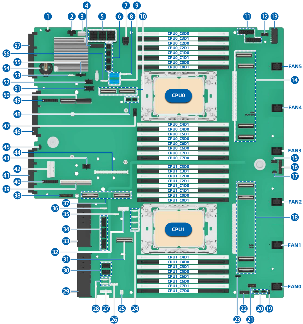
图 5-52 主板
