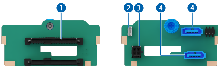
图 5-64 2 × 2.5 英寸硬盘 (2 × SAS/SATA) 背板
