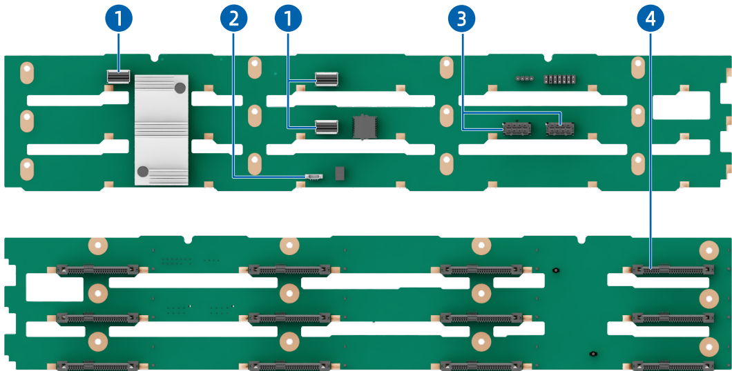
图 5-57 12 × 3.5 英寸硬盘配置 (12 × SAS/SATA) 背板
