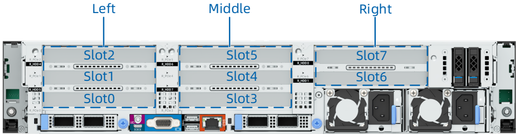
图 5-42 PCIe 插槽-8PCIe+2 M.2 配置
